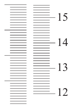
Vue partielle de l'échelle graduée 1/10°
